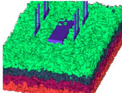
Simulation numérique du bourrage de ballast (une difficulté en plus ici : les contacts sont Non linéaires)
